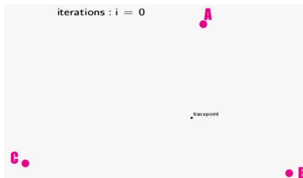
Рисунок 1. Построение стартовой точки O и треугольника ABC
