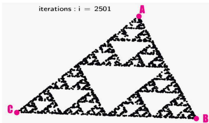
Рисунок 4. Построение спустя 2501 выброшенной точки
