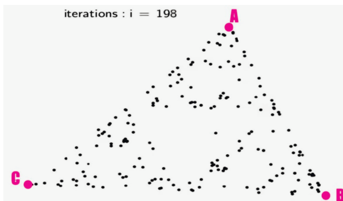
Рисунок 2. Построение спустя 198 выброшенных точек
