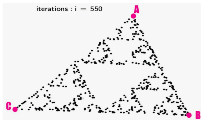
Рисунок 3. Построение спустя 550 выброшенных точек
